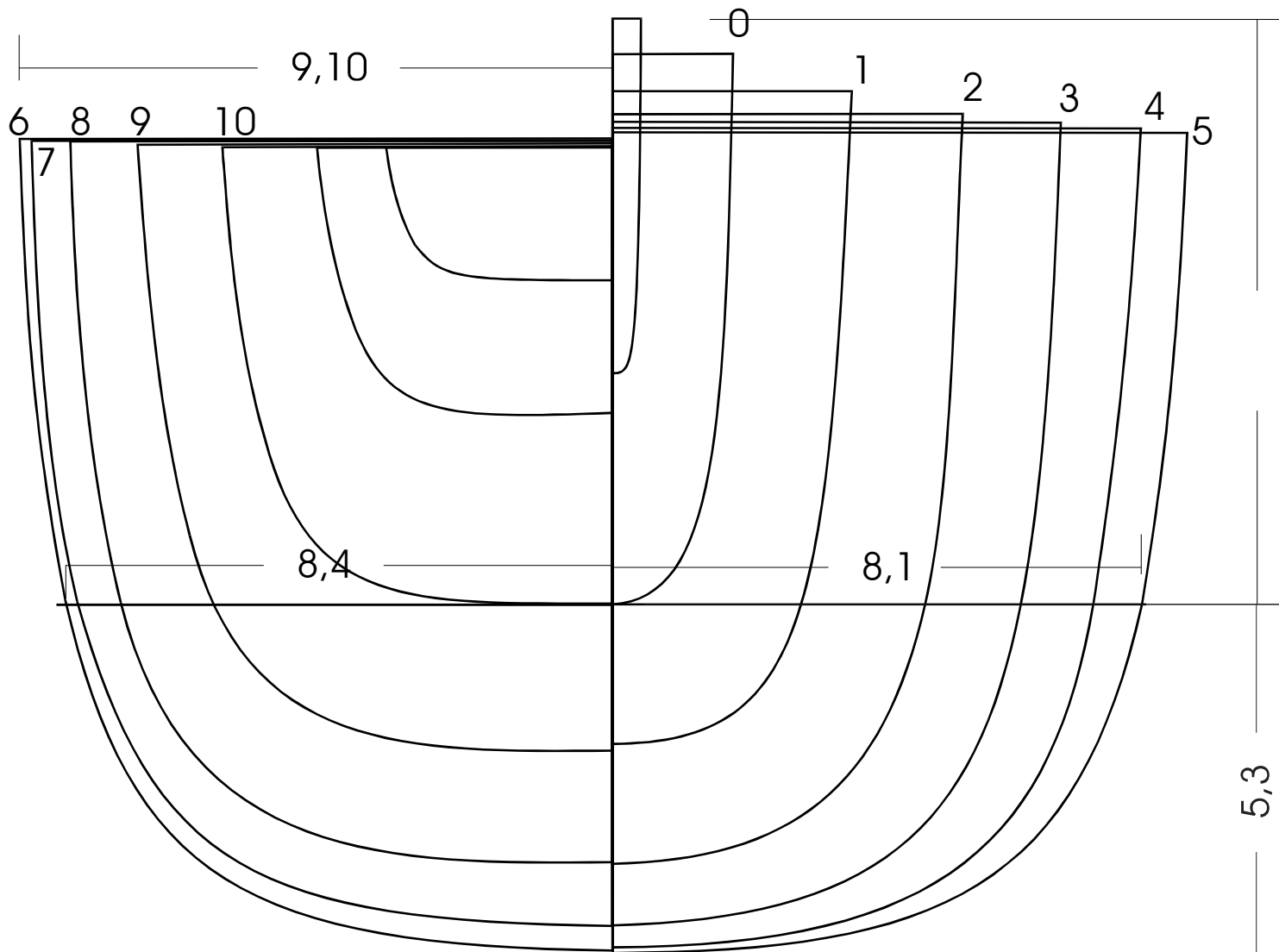
sezioni per modello RC di ALINGHI SUI-100 Scala 1 :1 compatibile con il Regolamento Safalero Cup
